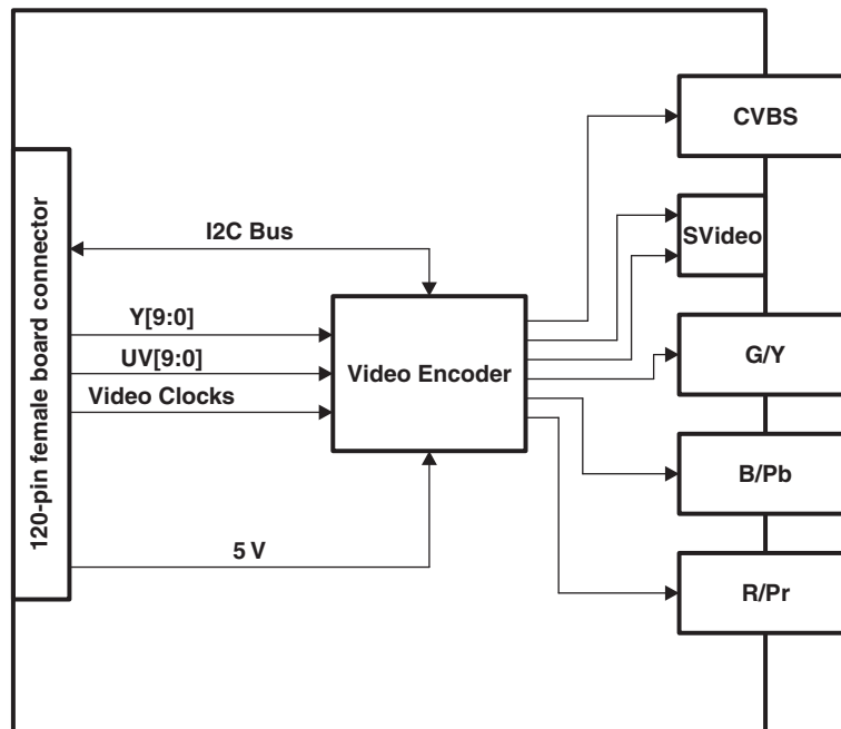
Figure 1-2. Encoder Module
