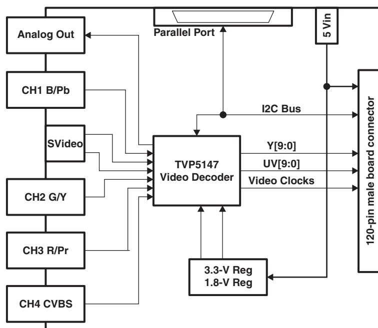
Figure 1-1. TVP5147 Module
