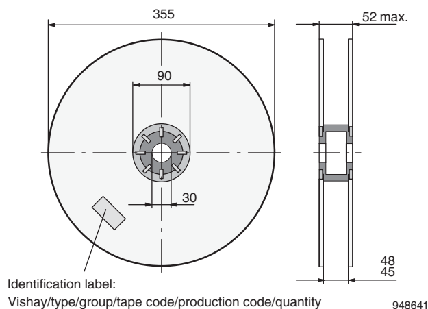
Fig. 20 - Reel
