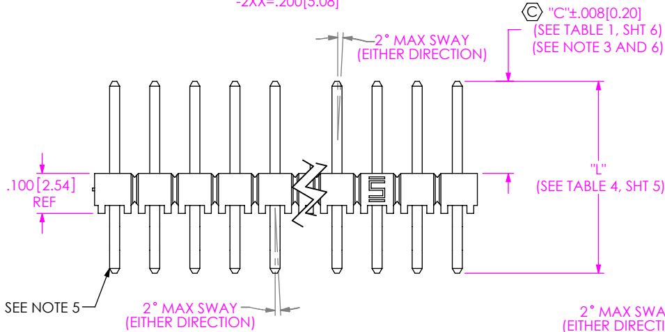
FIG 1 (TSW-1XX-XX-XX-S SHOWN)
