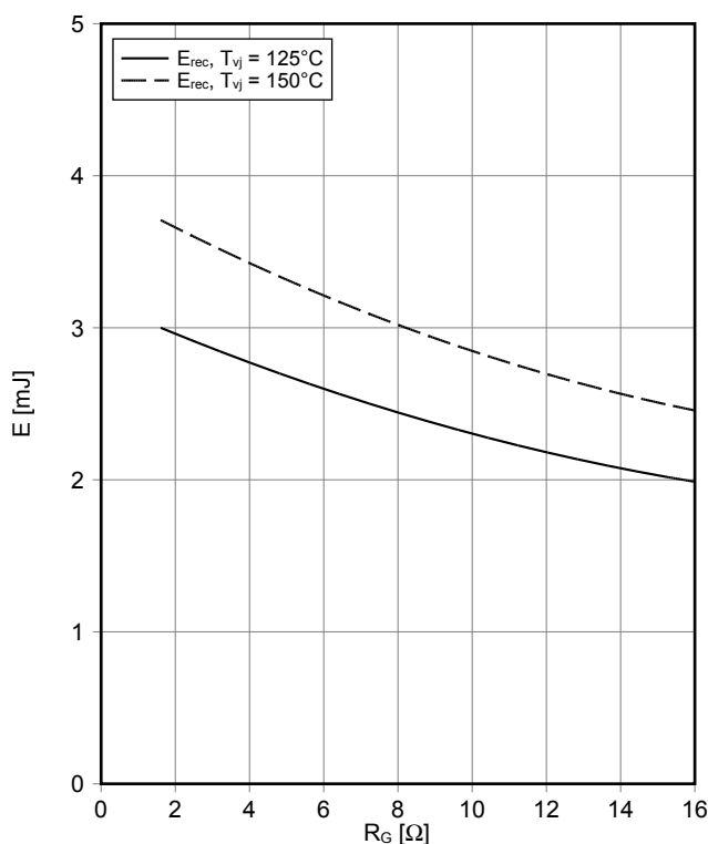
Schaltverluste Diode, Brems-Chopper (typisch) switching losses Diode, Brake-Chopper (typical) E_{rec} = f(R_G) I_F = 50 \text{ A} , V_{CE} = 600 \text{ V}
