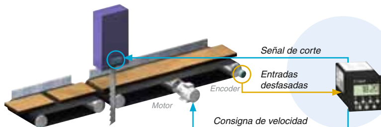
Corte a medida en máquina para madera
