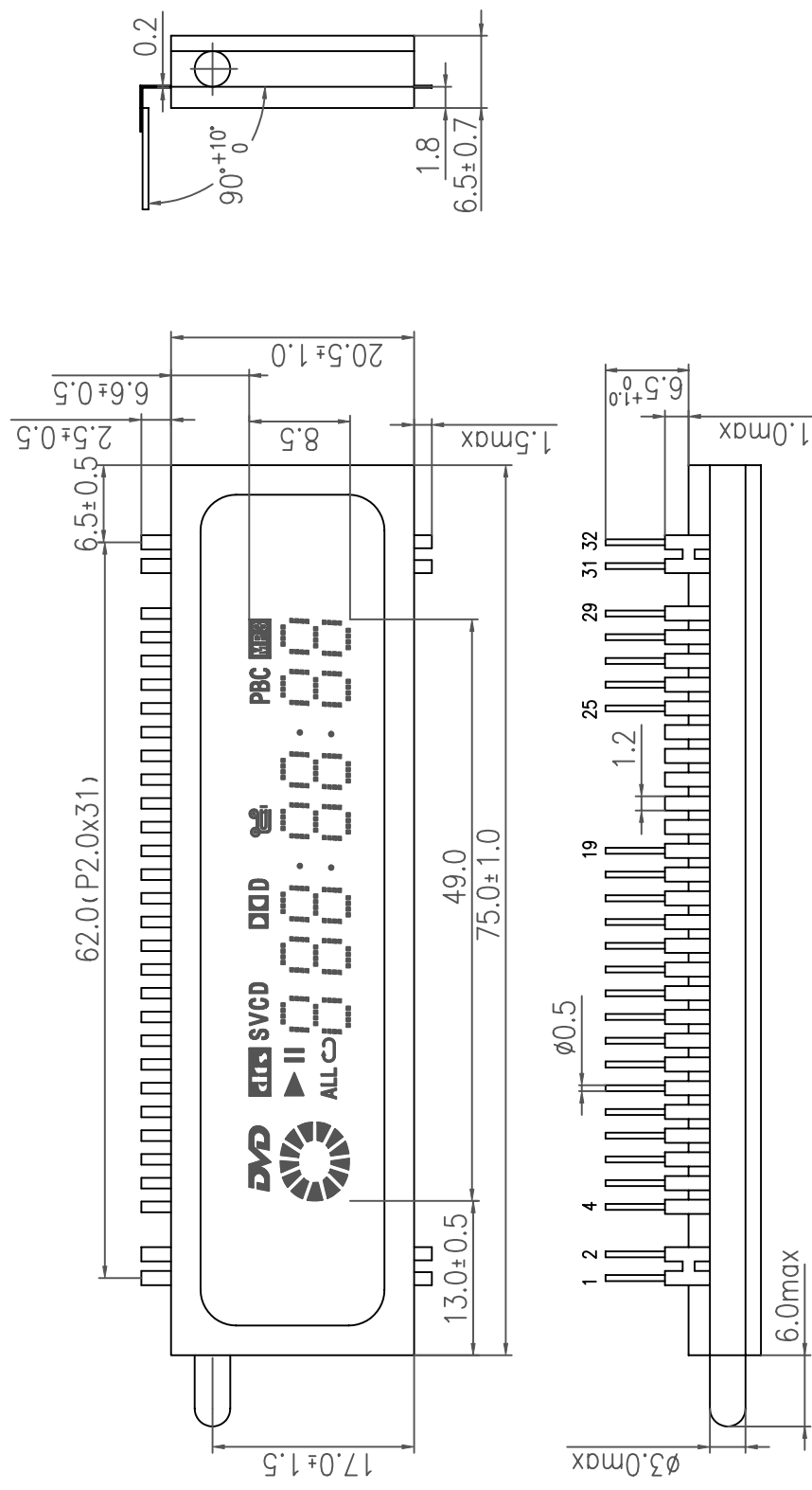
附图 1：外形图
