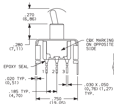
7101MD9_BE SPDT
