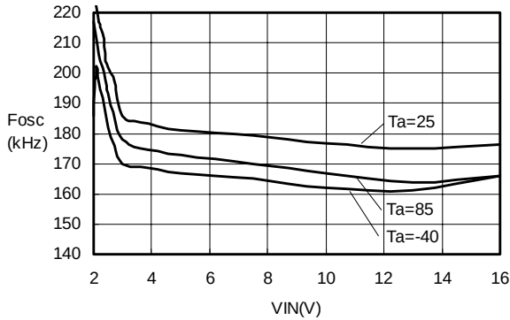
Fosc-VIN S-8520/21(Fosc:180kHz)
