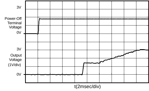
S-8521C30MC (Vin:9.0V)
