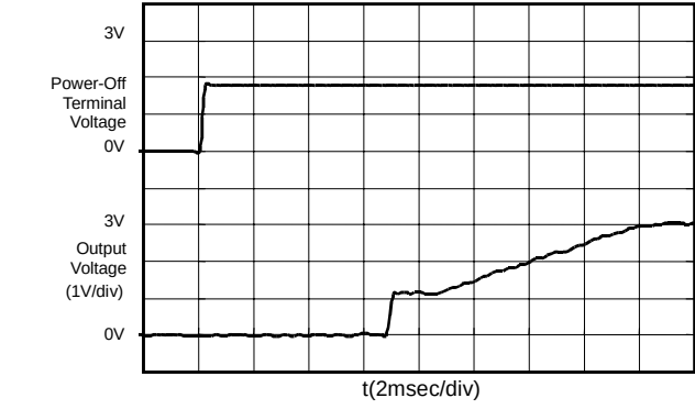
S-8521C30MC (Vin:3.6V)
