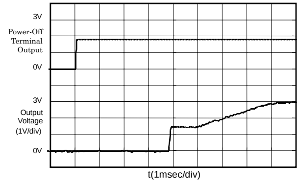
S-8520C30MC (Vin:9.0V)
