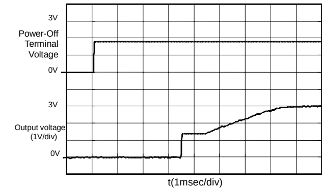
S-8521A30MC (Vin:3.6V)
