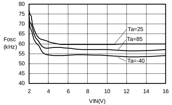
Fosc-VIN S-8520/21(Fosc:60kHz)
