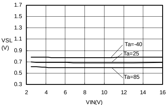
VSL-VIN S-8520/21
