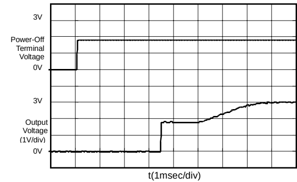
S-8521A30MC (Vin:9.0V)
