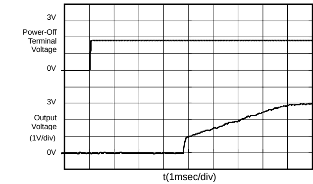
S-8520C30MC (Vin:3.6V)
