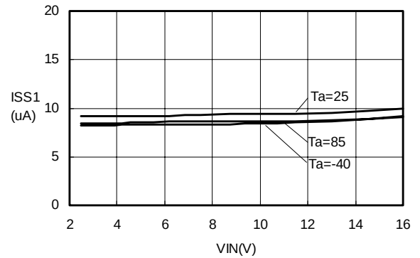
ISS1-VIN S-8520/21(Fosc:60kHz)
