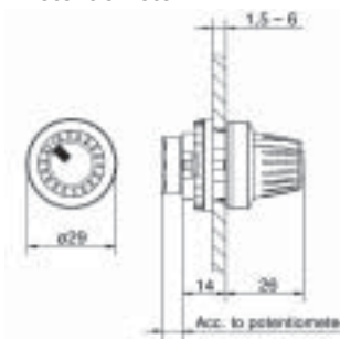
Potentiometer
