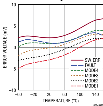
Handshake Voltage Error
