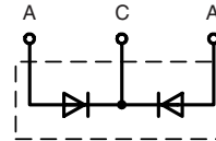
ISOPLUS 247™
