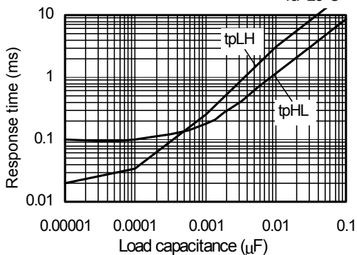
S-80960CN Ta=25°C
