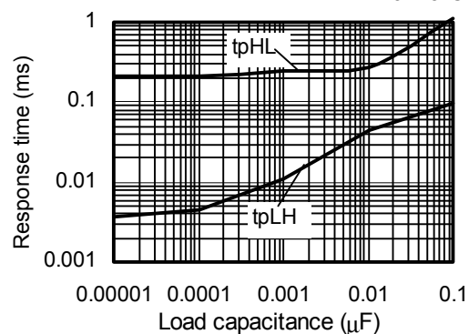
S-80914CL Ta=25°C
