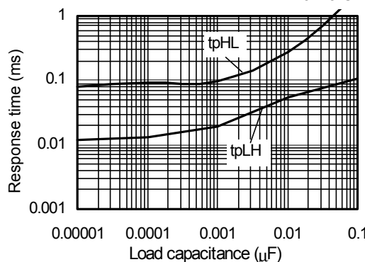
S-80960CL Ta=25°C
