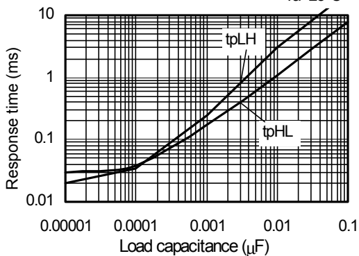
S-80960CN Ta=25°C
