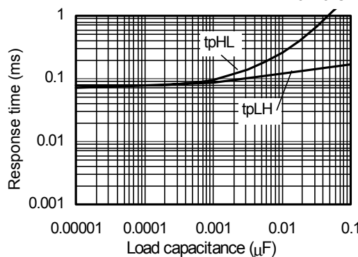
S-80960CL Ta=25°C
