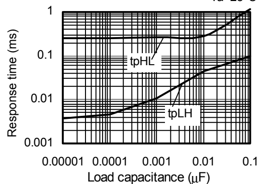
S-80915CL Ta=25°C
