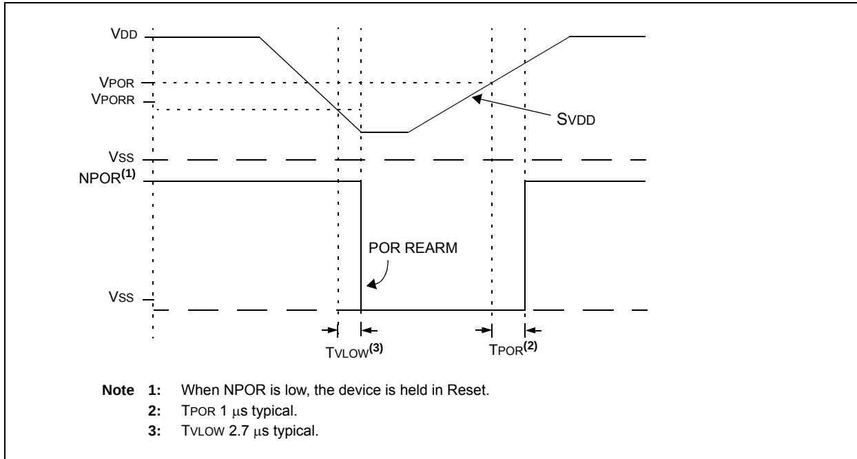
FIGURE 31-3: POR AND POR REARM WITH SLOW RISING V DD
