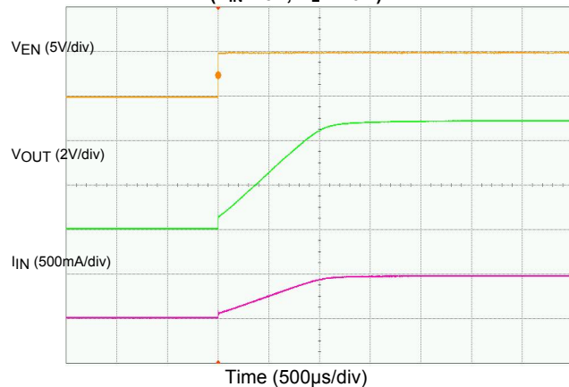
AP2281-1 Turn-On ( V_{IN} = 5V , R_L = 10\Omega )
