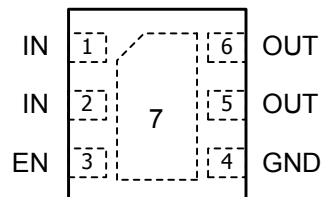
U-DFN2018-6
