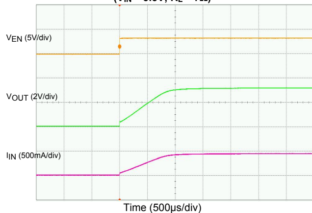
AP2281-1 Turn-On ( V_{IN} = 3.3V , R_L = 7\Omega )
