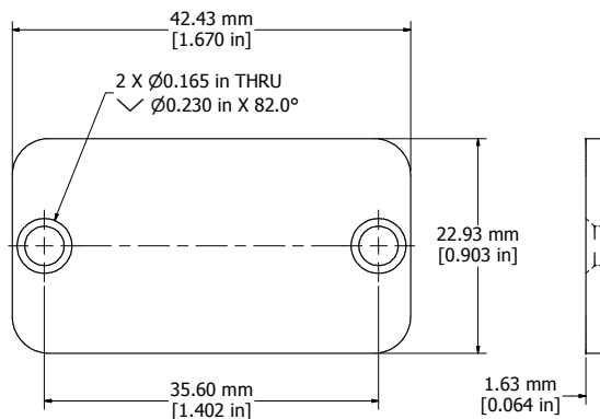
ENDPLATE
