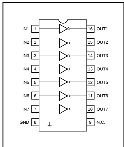
BA6250 / BA6250F
