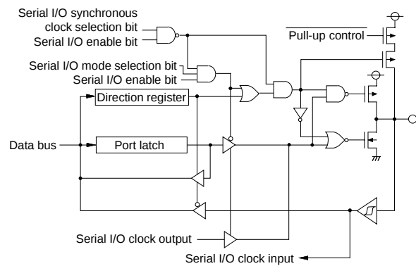
(4) Port P31
