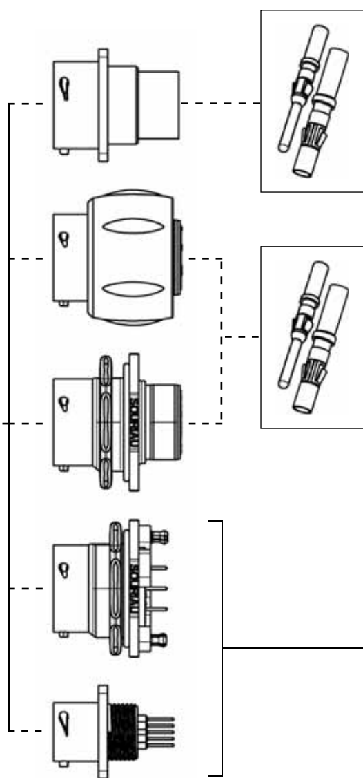
Receptacle
