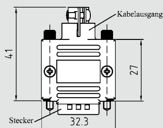
Maße für 9-polige Hauben / Dimensions for size 9 hoods
