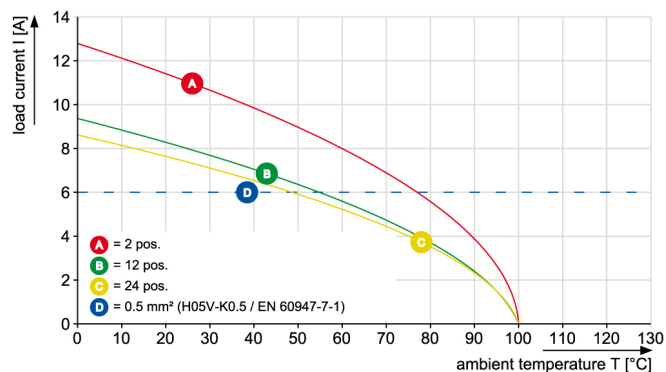
BL 3.50/./90 & /270 - SL 3.50/./90
