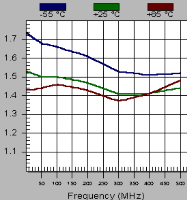
TM6511 Output VSWR
