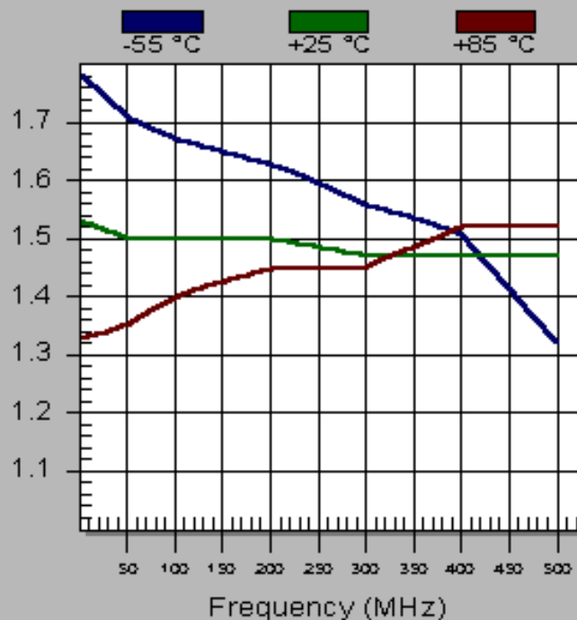
TM6511 Input VSWR
