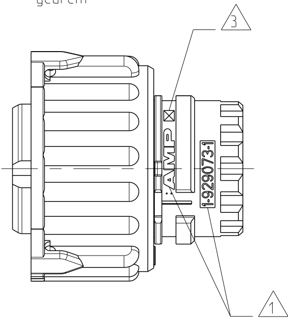
VIEW B ROTATED Ansicht B gedreht
