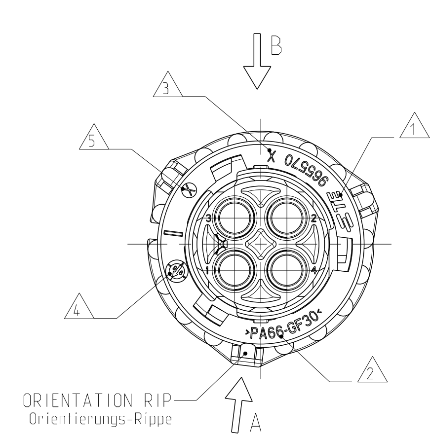
COUPLING RING IN PRE-LOCKED POSITION (FITTING POSITION WITH PIN HOUSING) Kupplungsring in Vorraststellung (Fuegeposition mit Stiftgehaeuse)
