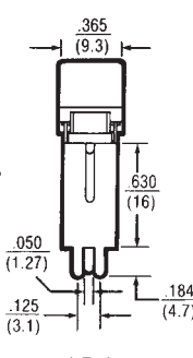
1 Pole
