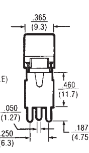
1 Pole
