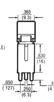
1 Pole
