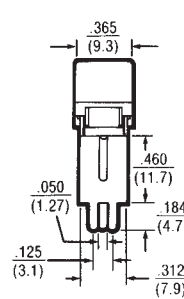
1 Pole
