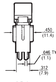
2 Pole
