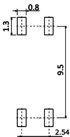
Fig. 13.1 Unit: mm
