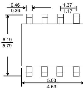
SOIC-8
