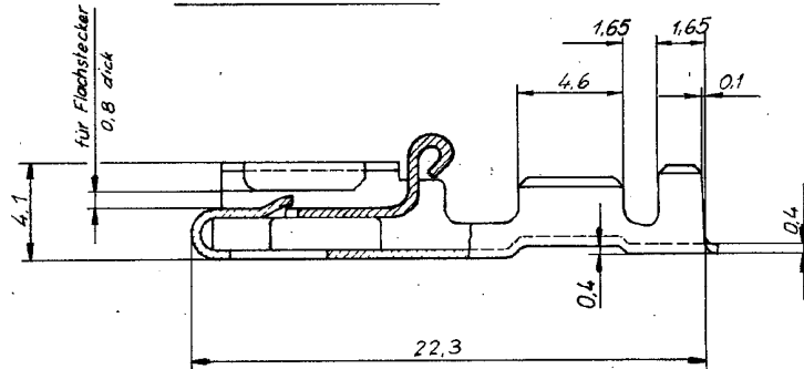
Teilschnitt: C - C
