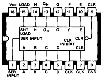
B117 SN74166N Shift register
