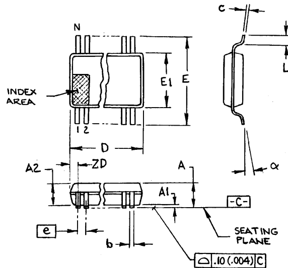
150 mil SSOP
