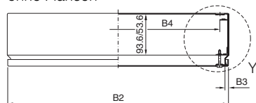
ohne Flansch
