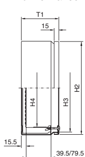
ohne Flansch
