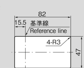
パネル穴明け寸法 (A-542-4-R) Panel drilling dimensions
