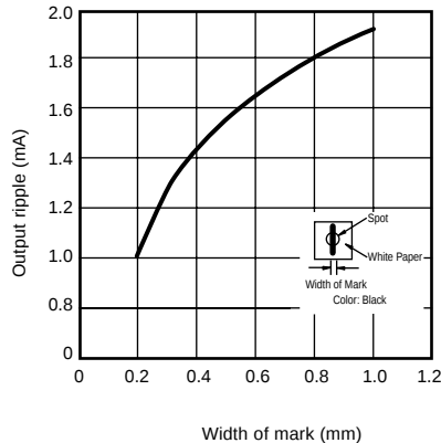
Mark Sensor Type E3SA-VSRC43A
