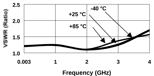
RF1 - RF4 On VSWR Temp. Variation
