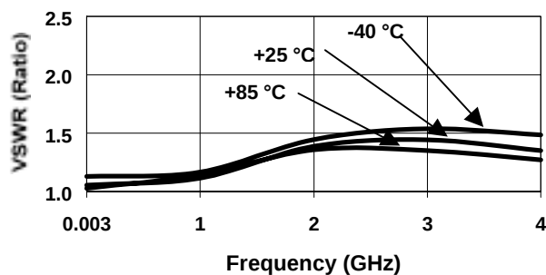
RF1 - RF4 Off VSWR Temp. Variation
