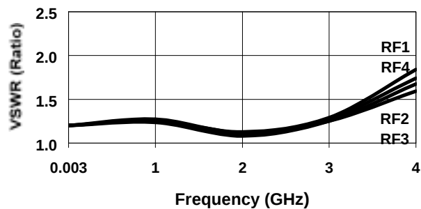
RF1 - RF4 On VSWR @ 25 °C
