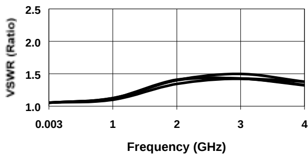
RF1 - RF4 Off VSWR @ 25 °C
