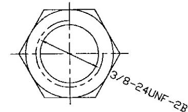
JAM NUT
