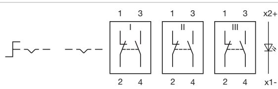
Wiring diagram 279
