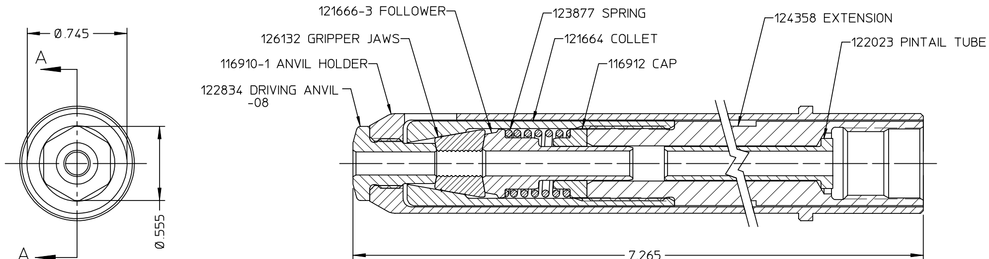
SECTION A-A
