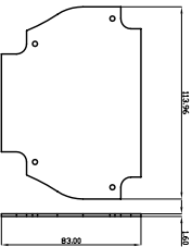
BOTTOM-PCB
