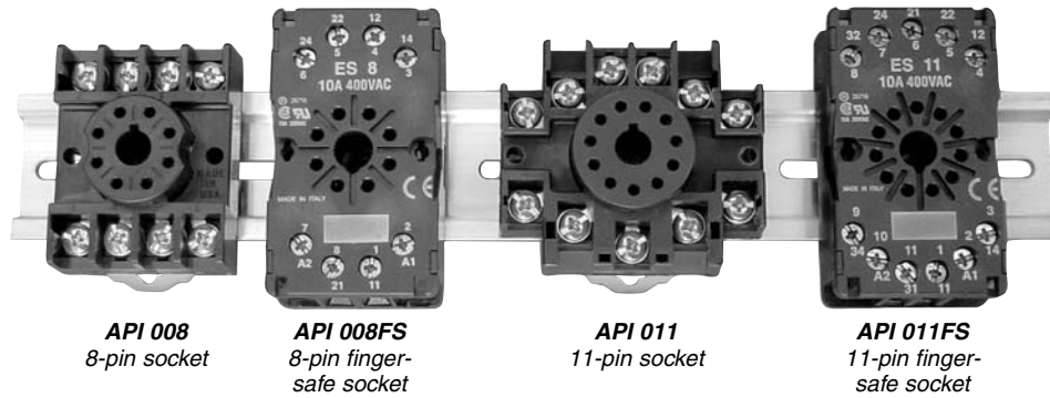
API TK36 DIN Rail
