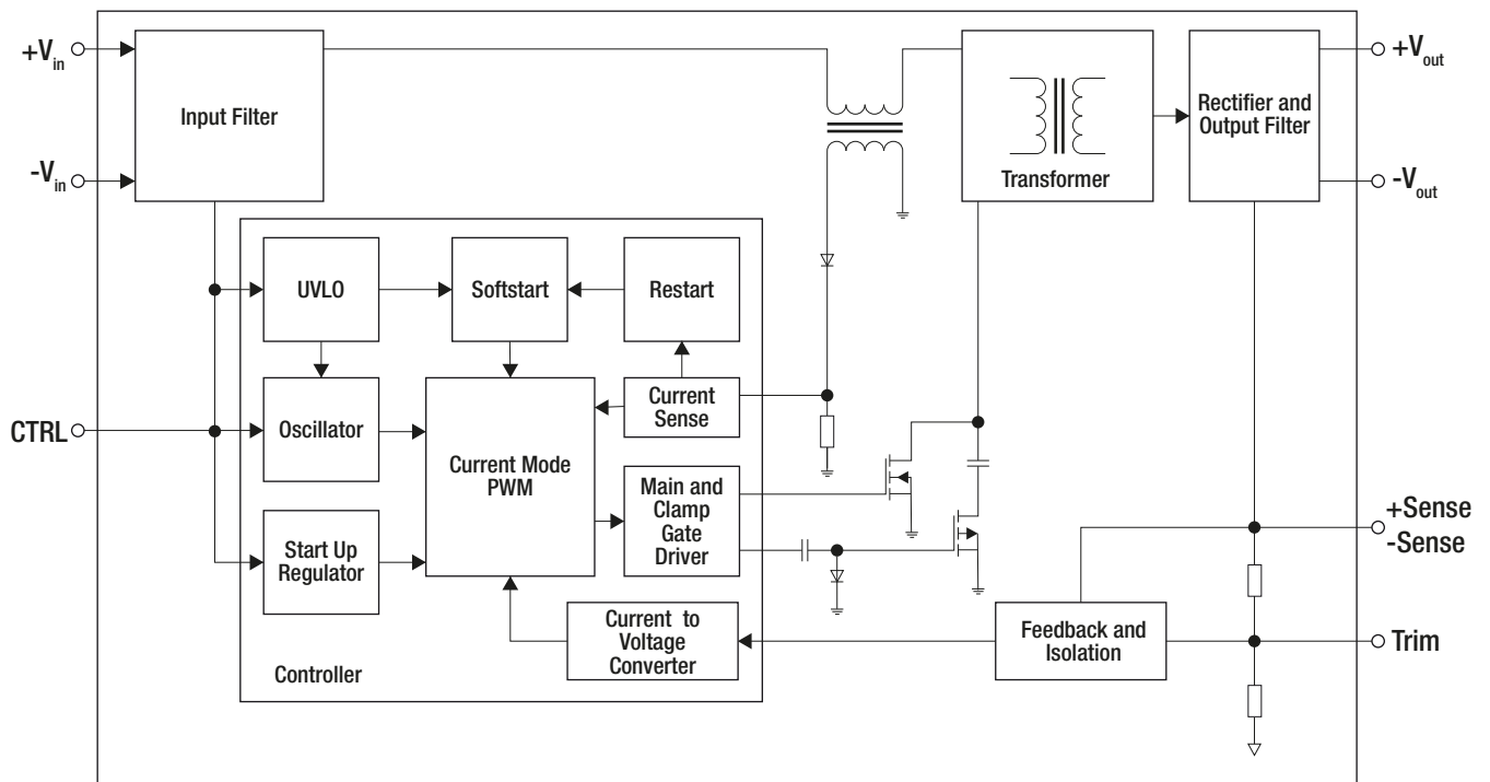
BLOCK DIAGRAMM
