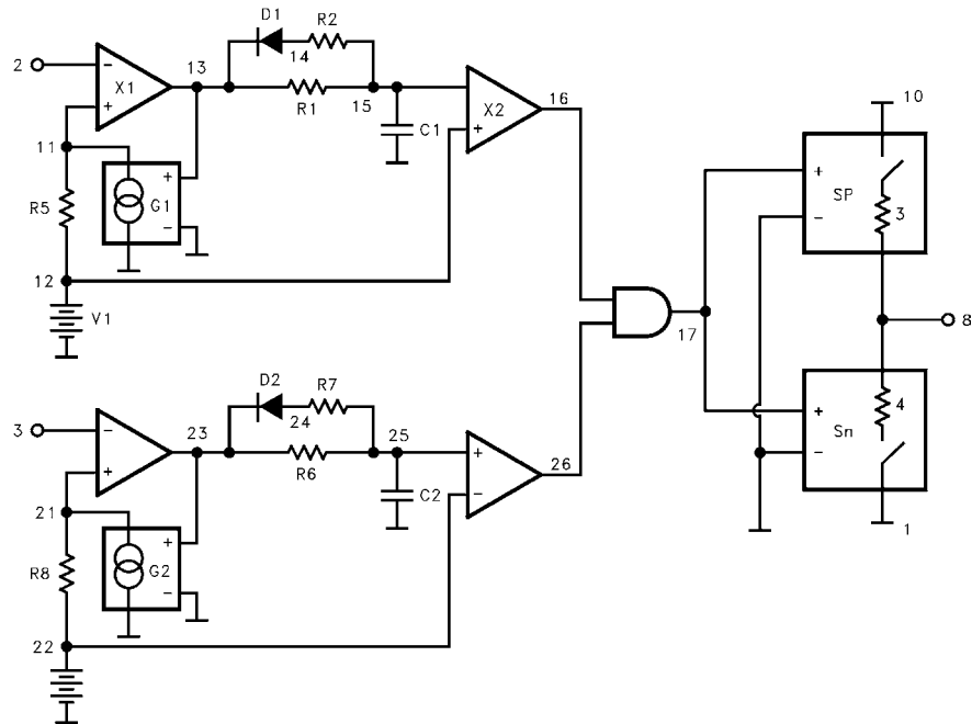
EL7243 Macromodel
