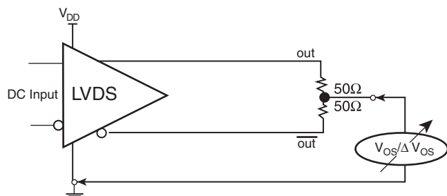
V_{OS} SETUP
