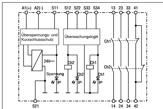
FIG. 38: RELAIS-BLOCKSCHALTBIKD
