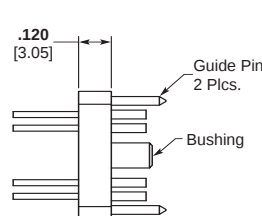
Receptacle
