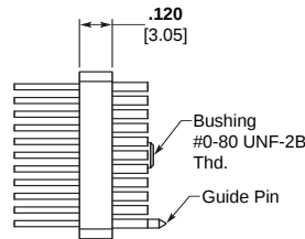
Receptacle
