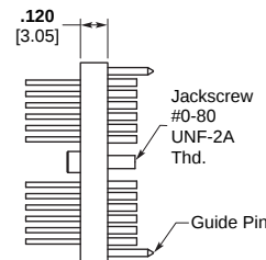
Receptacle
