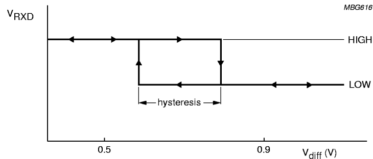
Fig.5 Hysteresis.
