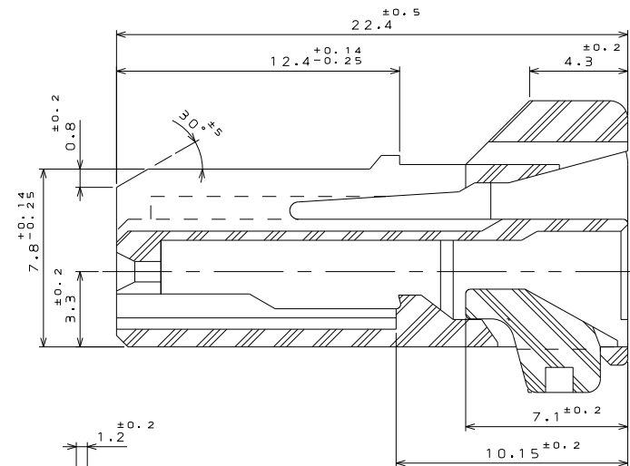
断面 A-A (尺度 5:1)
