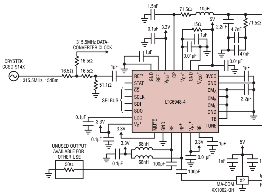
Generating a 12GHz LO Signal
