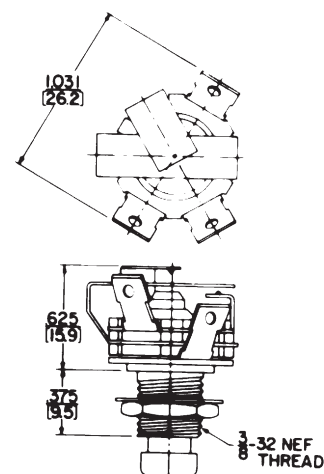
SPDT 1-C
