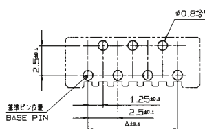
基板穴明け寸法 (コネクタ接合側) MOUNTING LAYOUT (CONN. MOUNTING SIDE) (適用基板厚 セ=1~1.6mm) (BOARD T.H.K 1~1.6mm)
