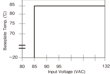
PF1000A-360 (At 85°C Baseplate Temp.)
