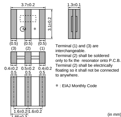
CSACV_X_Q 14.70-70.00MHz
