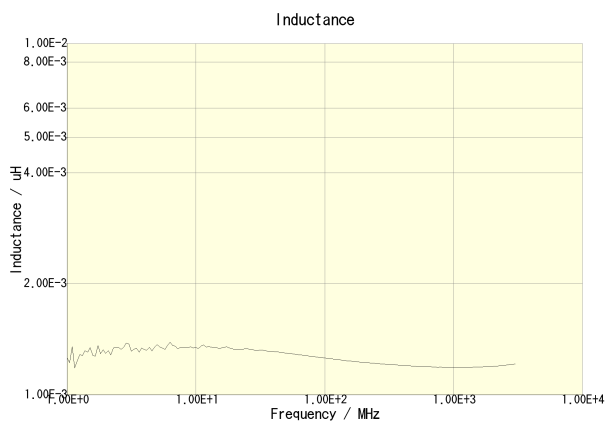
MLG1005S1N3ST000
