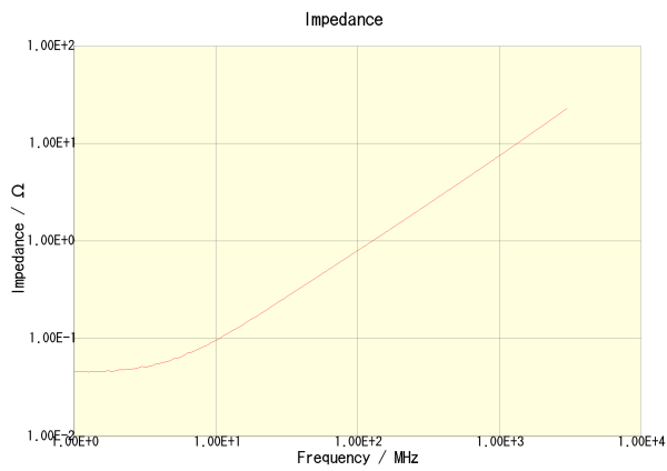
MLG1005S1N3ST000
