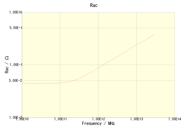
MLG1005S1N3ST000
