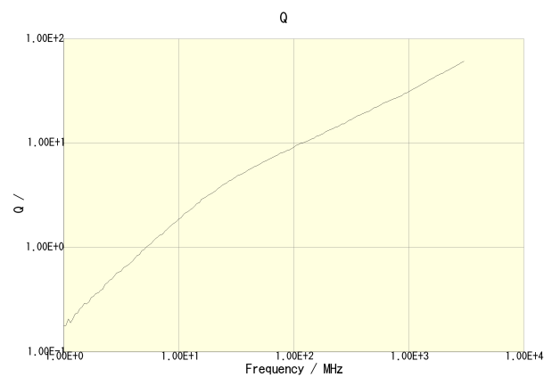
MLG1005S1N3ST000
